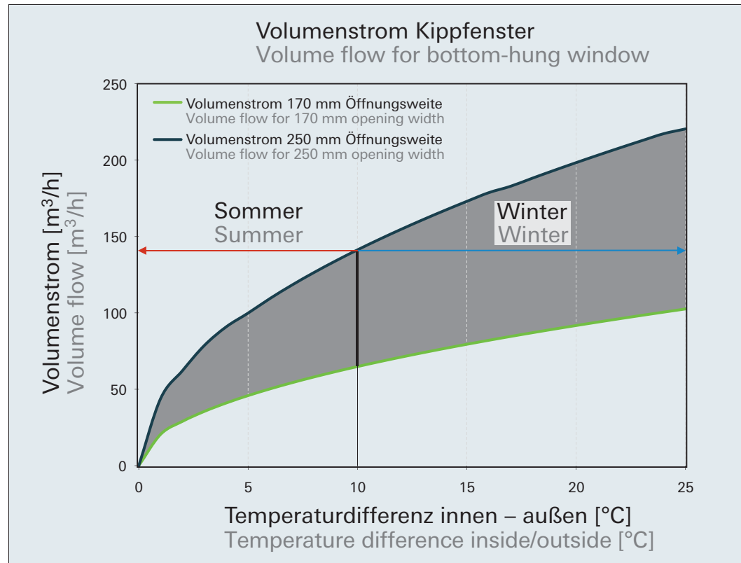
Vergleich Fensterluftwechsel Kippfenster Schüco TipTronic und Schüco TipTronic SimplySmart Comparison of air exchange in Schüco TipTronic and Schüco TipTronic SimplySmart bottom-hung windows
